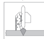
Altura do reforço da face da solda
